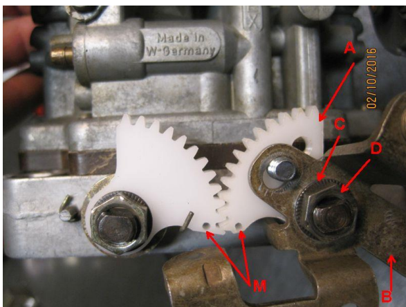
Bild 11: Primärsegment „A“ auf Primärwelle aufschieben. Die beiden Markierungsbohrungen „M“ der Segmente stehen gegenüber (Detail „M“ im Bild 11)
